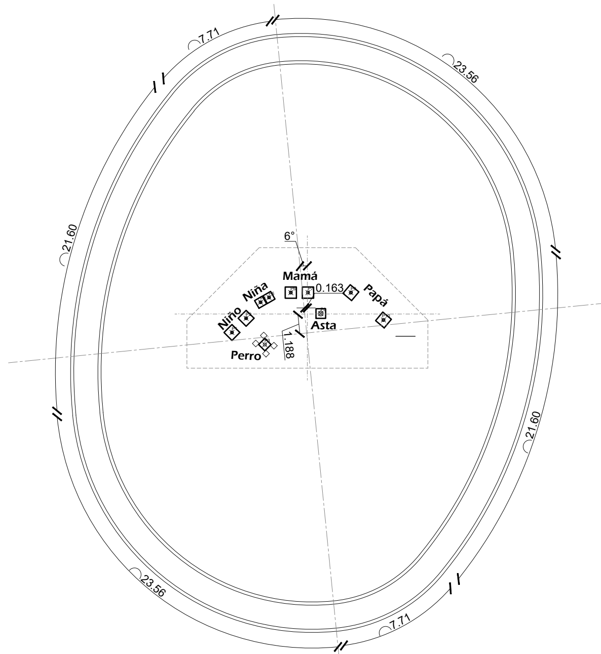
01 PLANTA DE UBICACION DE FIGURAS ESCALA= s/e
